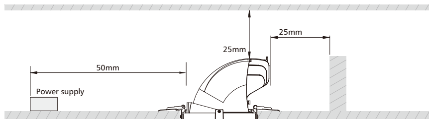
Fig 1: Espacement d'installation / Installation Spacing
