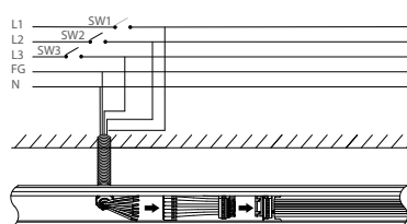
Cablage pour 3 circuits avec le 5 files / Wire diagram of triple circuits function
